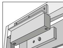
"L" Bracket: in narrow profiles/ Soporte "L": En perfiles estrechos
